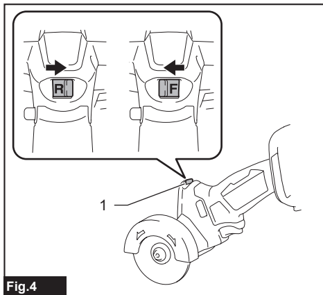
Fig.4 ► 1. Interruptor de reversión de rotación
